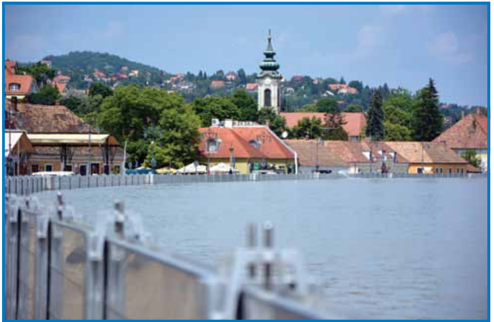
Mobil árvízvédelmi fal védte meg Szentendre belvárosát 2013-ban
